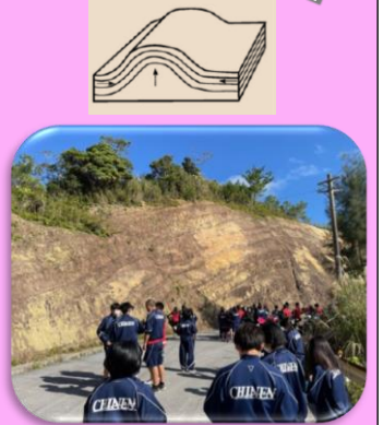
名護市底仁屋にて 嘉陽層の褶曲観察
